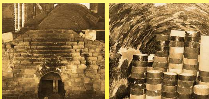
Four Dragon traditionnel chinois (龙窑 Long Yao), vue de la bouche d'alimentation et méthode de remplissage avec des porcelaines électriques (collection privée).
